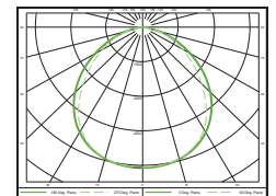
CLF24-VH1-C-UV / Lumens: 15370
